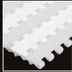
25-808F Superficie cerrada con módulos de alta fricción. Para transportes en plano inclinado. Fácil de limpiar
